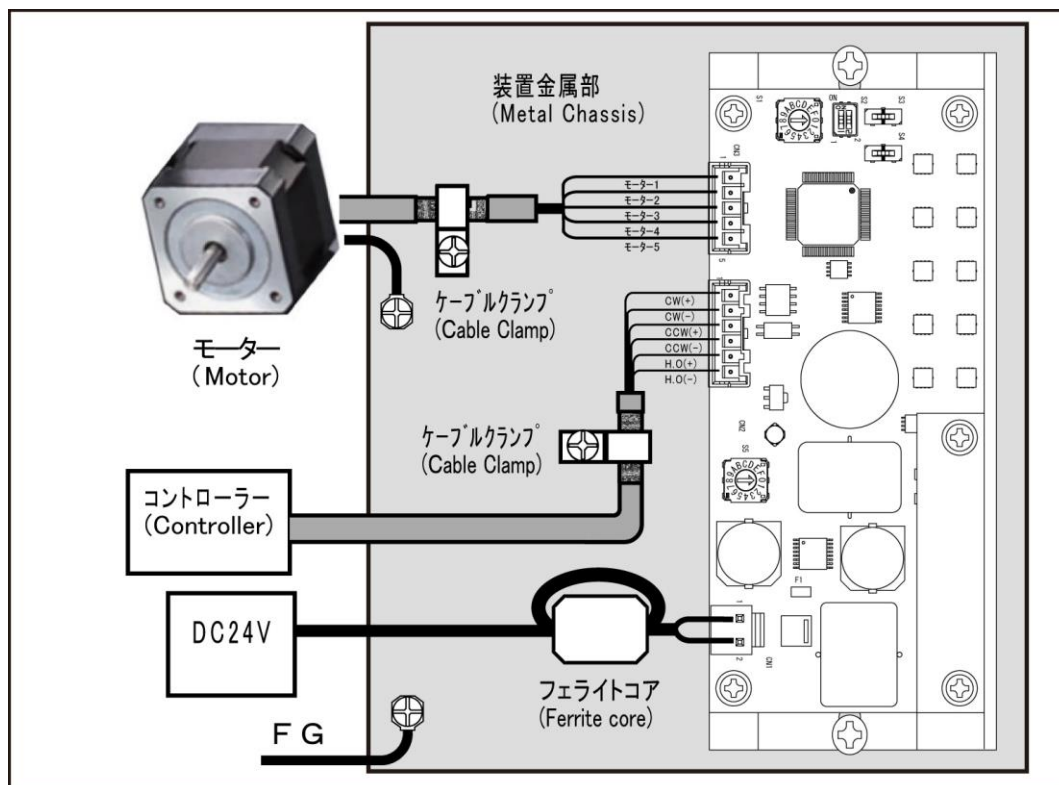
モーター、ドライバの設置、配線例4
